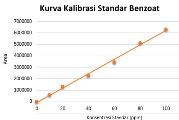
Gambar 1. Kurva Kalibrasi Benzoat
