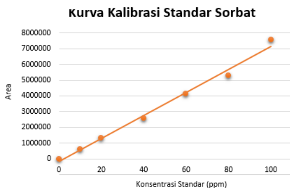
Gambar 2. Kurva Kalibrasi Sorbat
